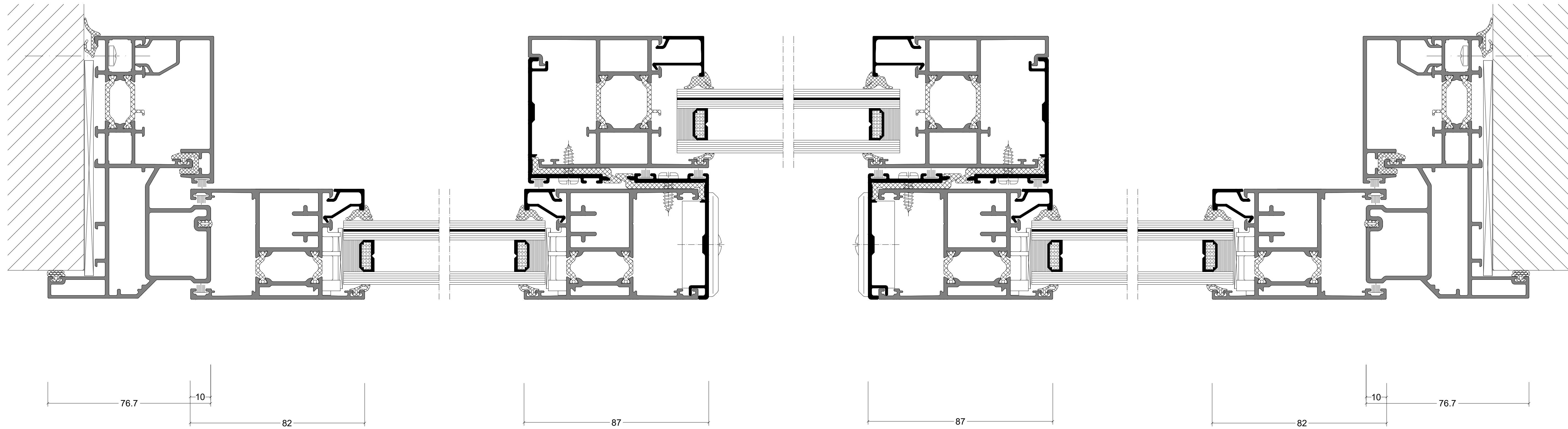
BOUWKUNDIGE AANSLUITINGEN 1:1
