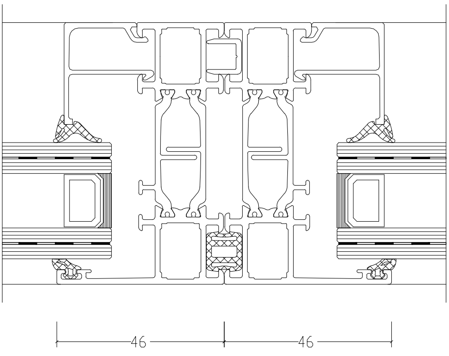
Verborgen koppeling
