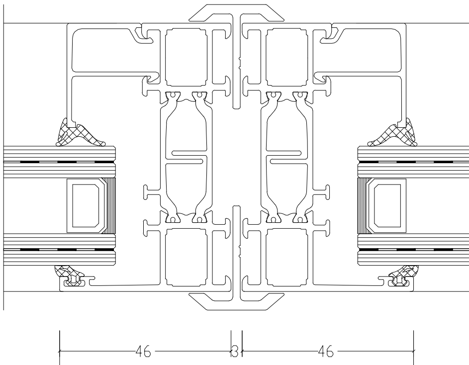
Losse koppeling
