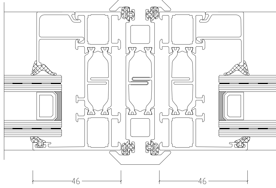
Vlakke koppeling
