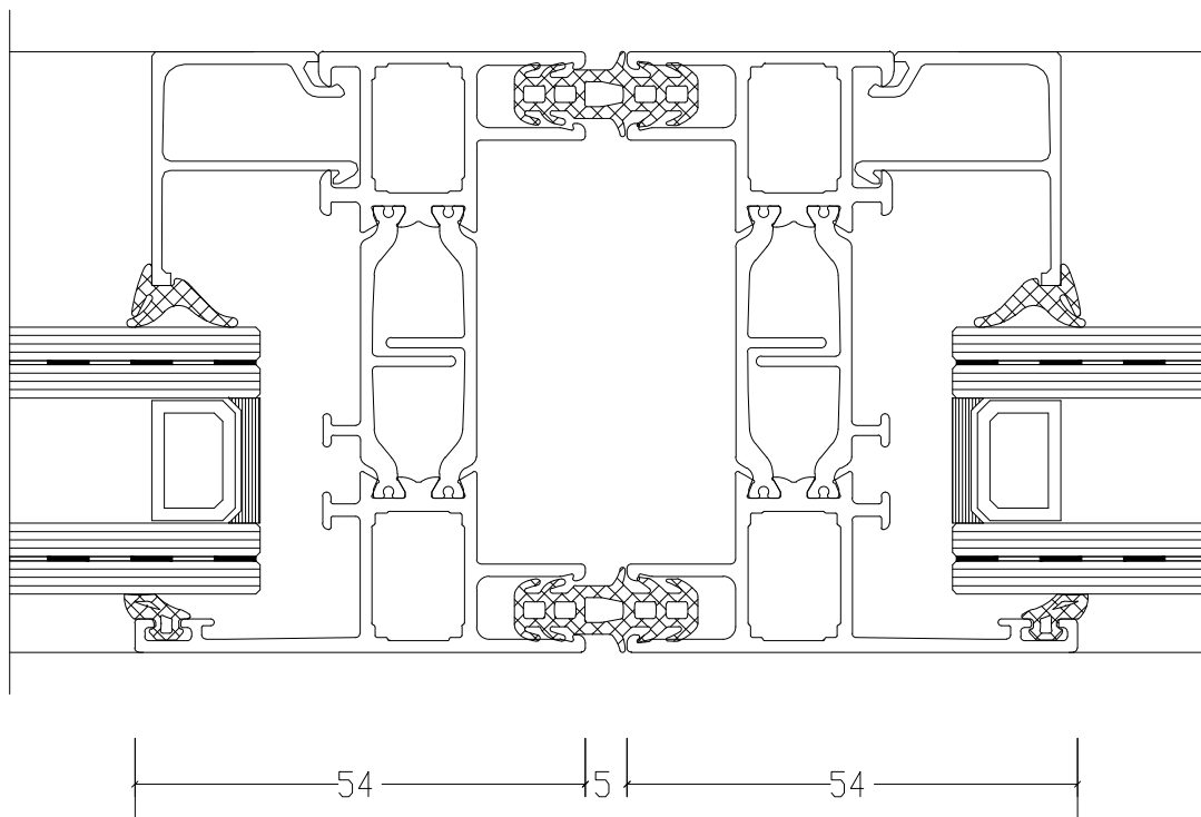
Dilatatie koppeling
