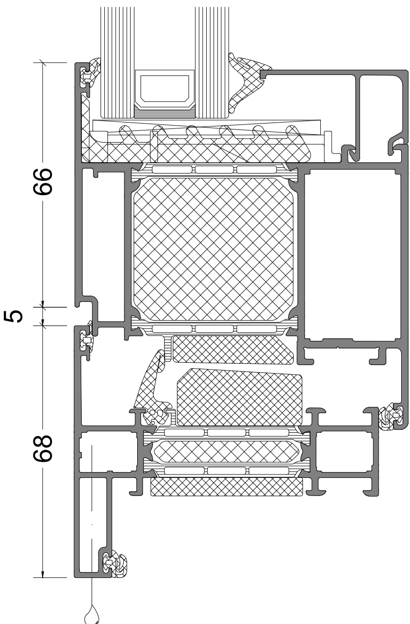
VERBORGEN WATERAFVOER
