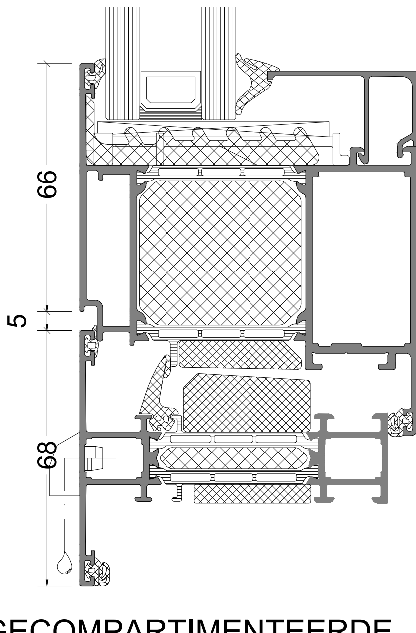
GECOMPARTIMENTEERDE WATERAFVOER
