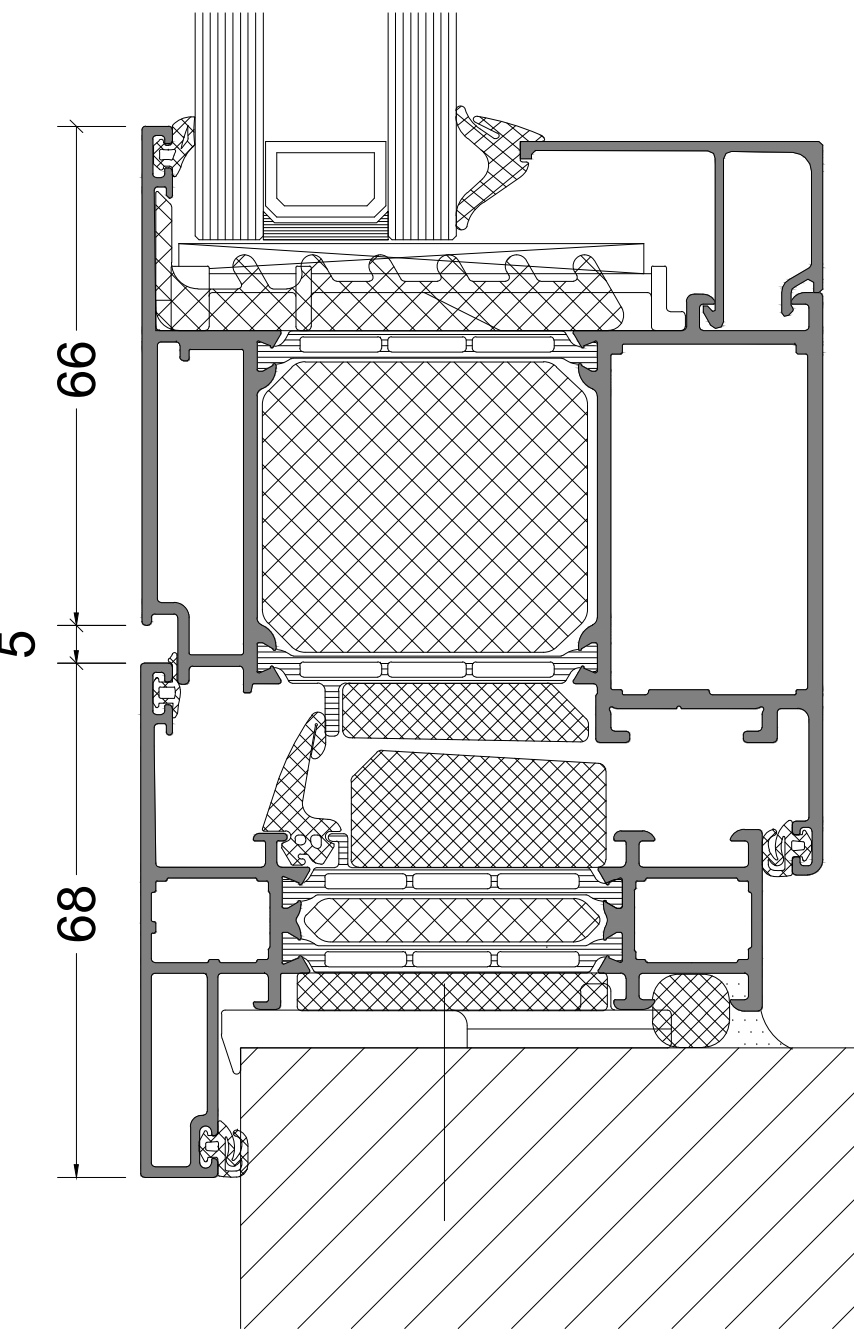
AANSLUITING ONDER
