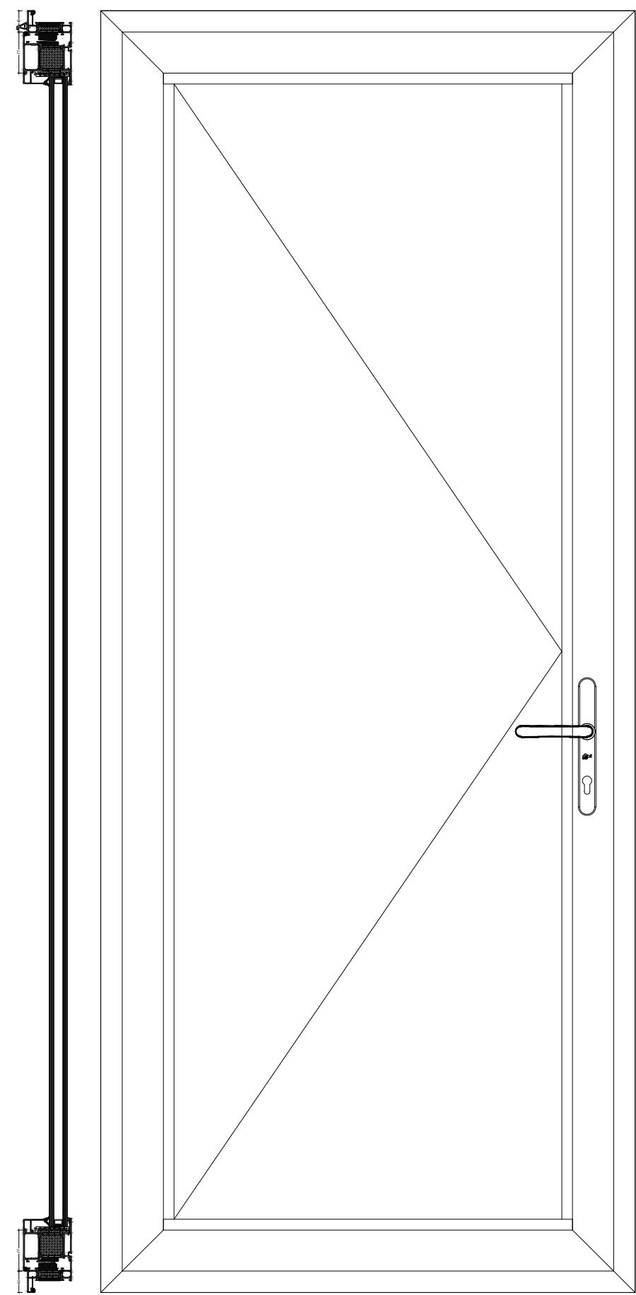
OPDEKDEUR BINNENDRAAIEND
