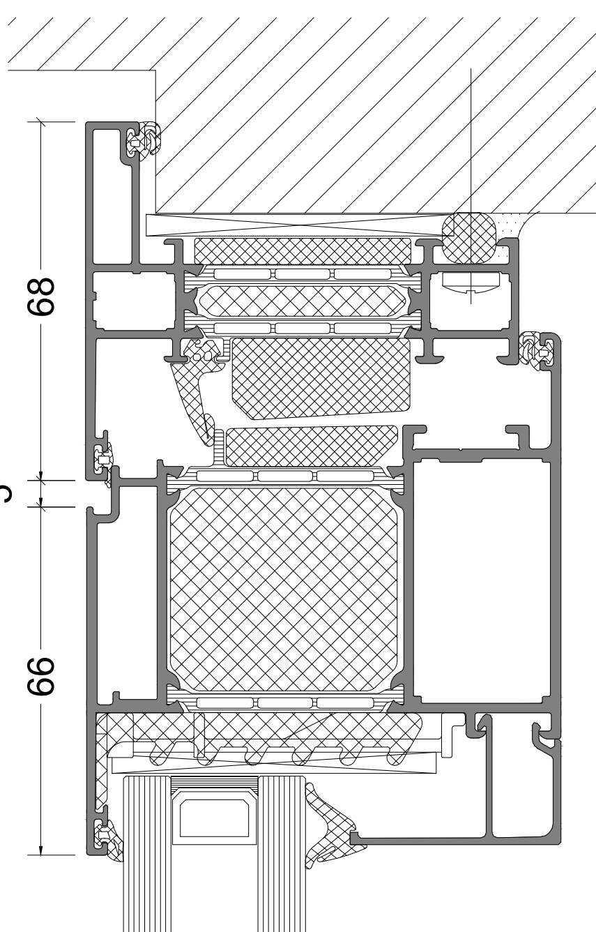
AANSLUITING BOVEN
