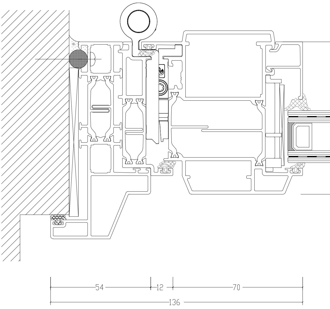
AANSLUITING ZIJ
