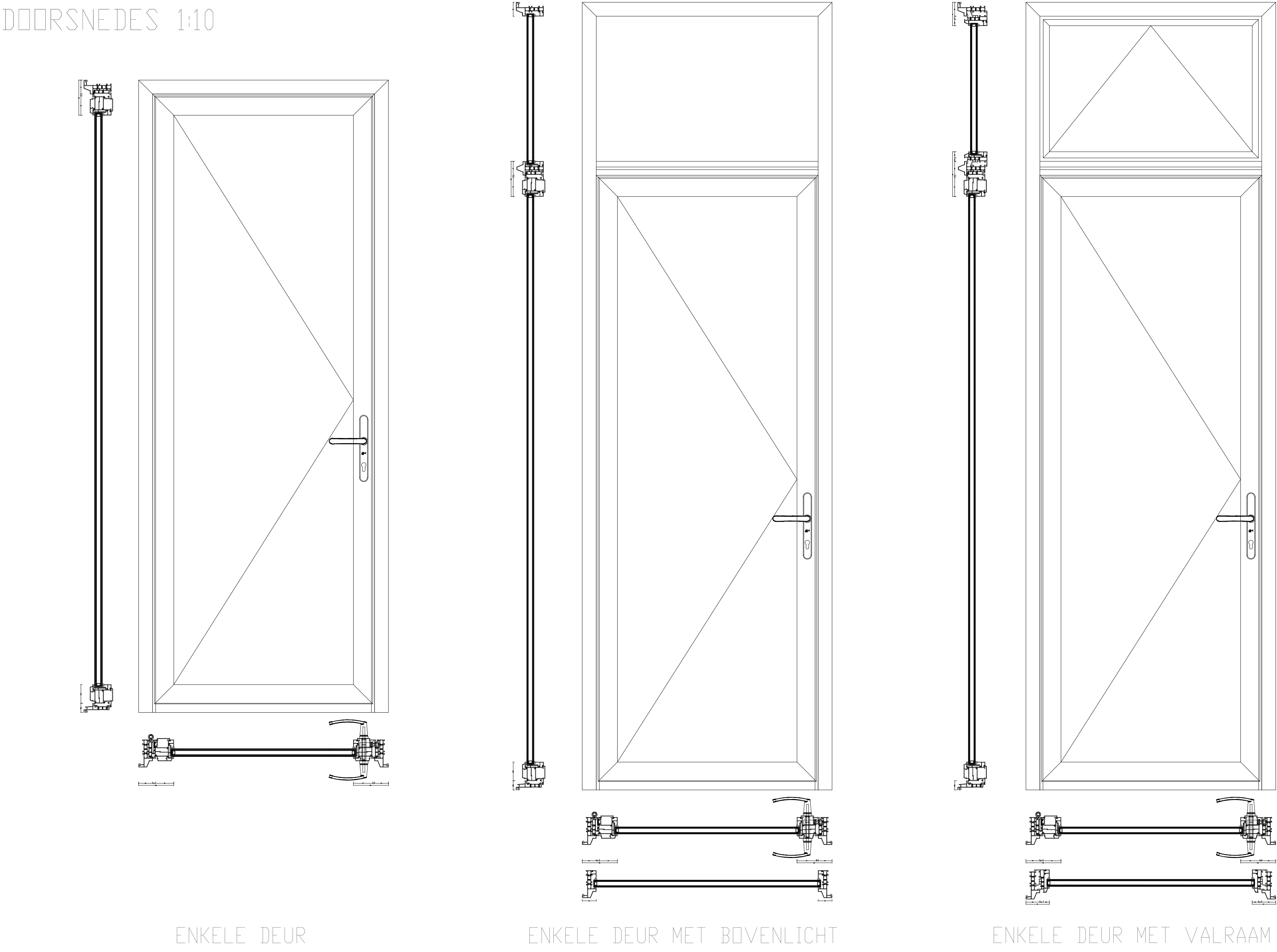
ENKELE DEUR
