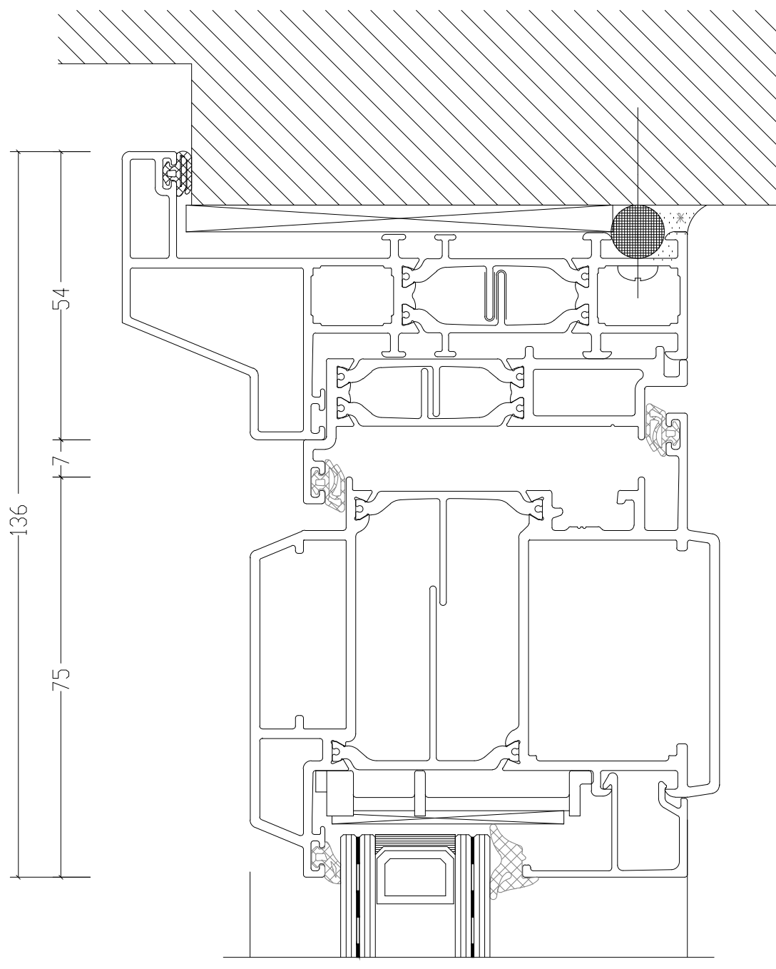
AANSLUITING BOVEN
