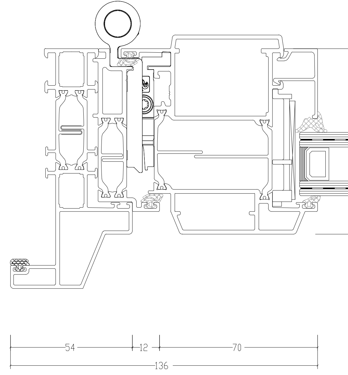
DUBBEL GLAS
