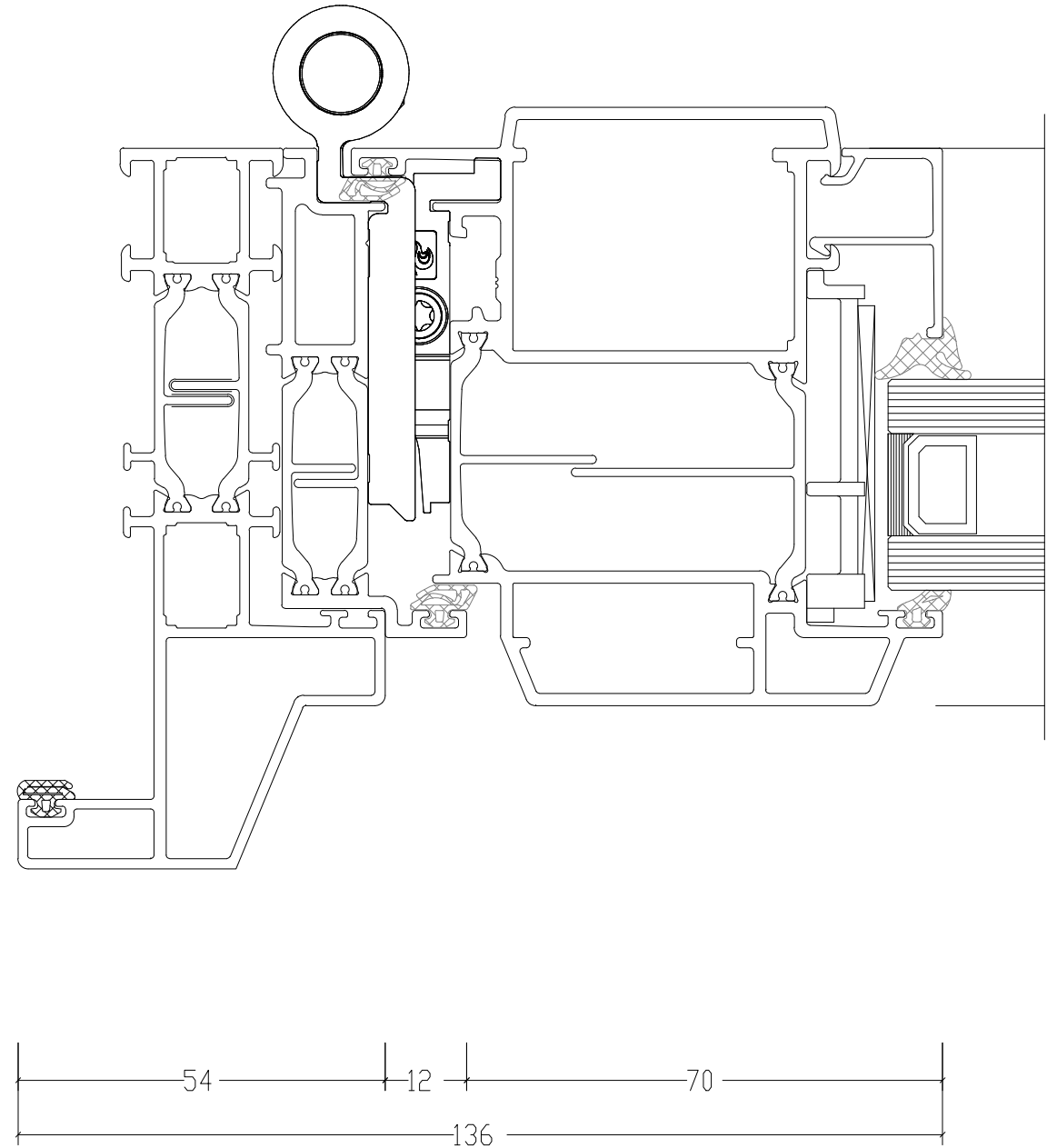
DUBBEL GLAS
