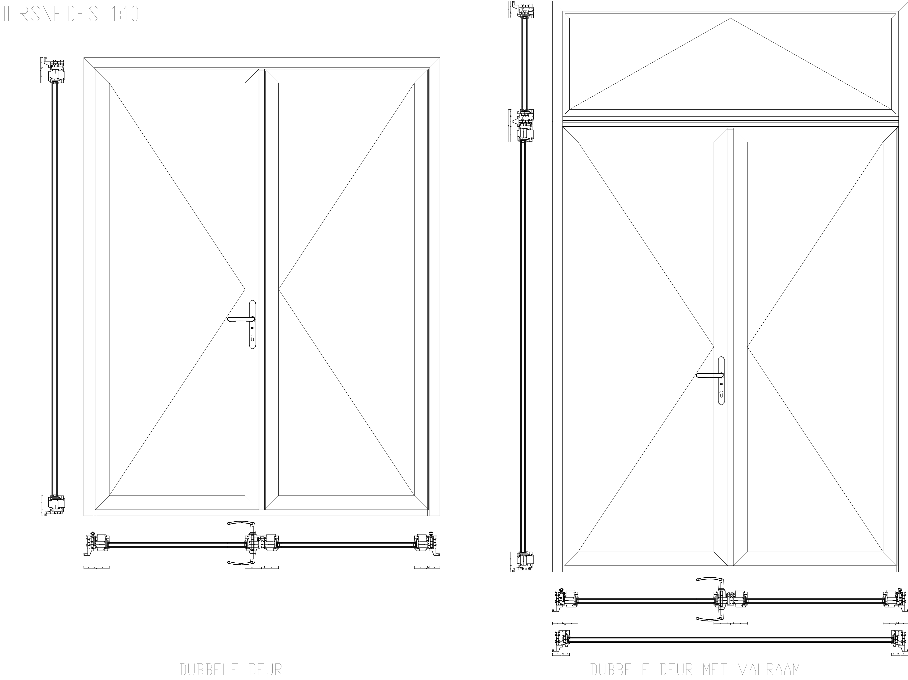
DUBBELE DEUR
