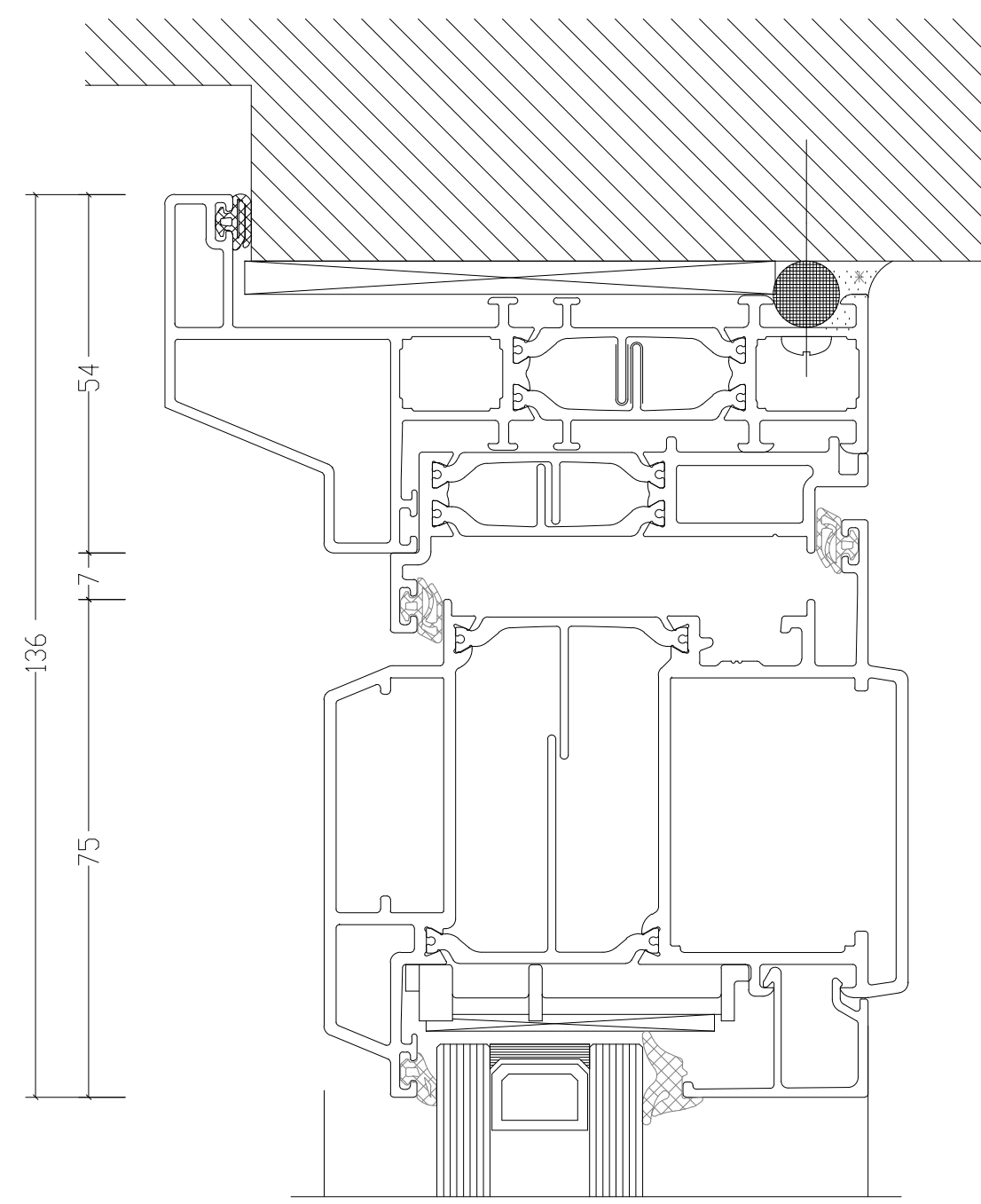
AANSLUITING BOVEN
