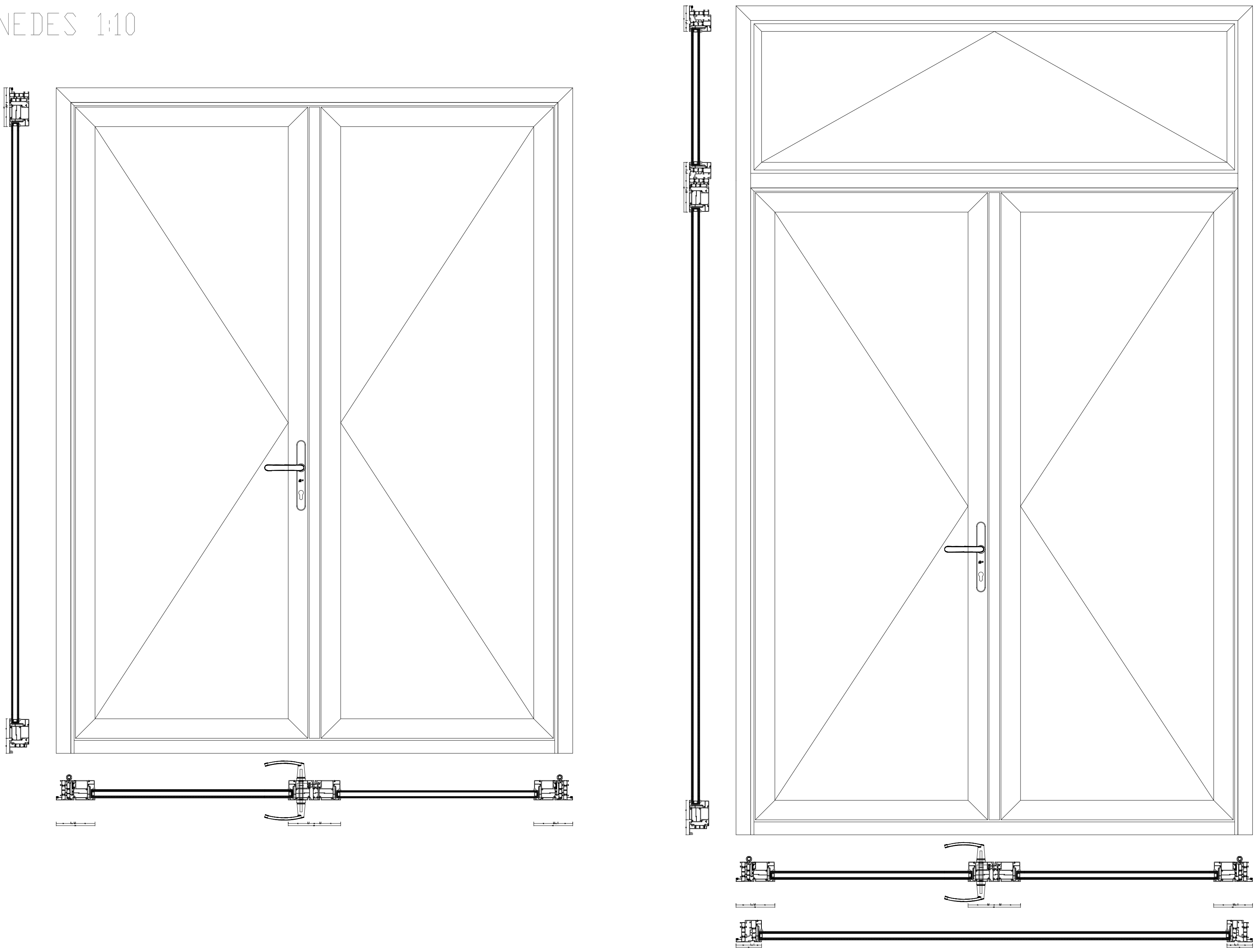
DUBBELE DEUR
