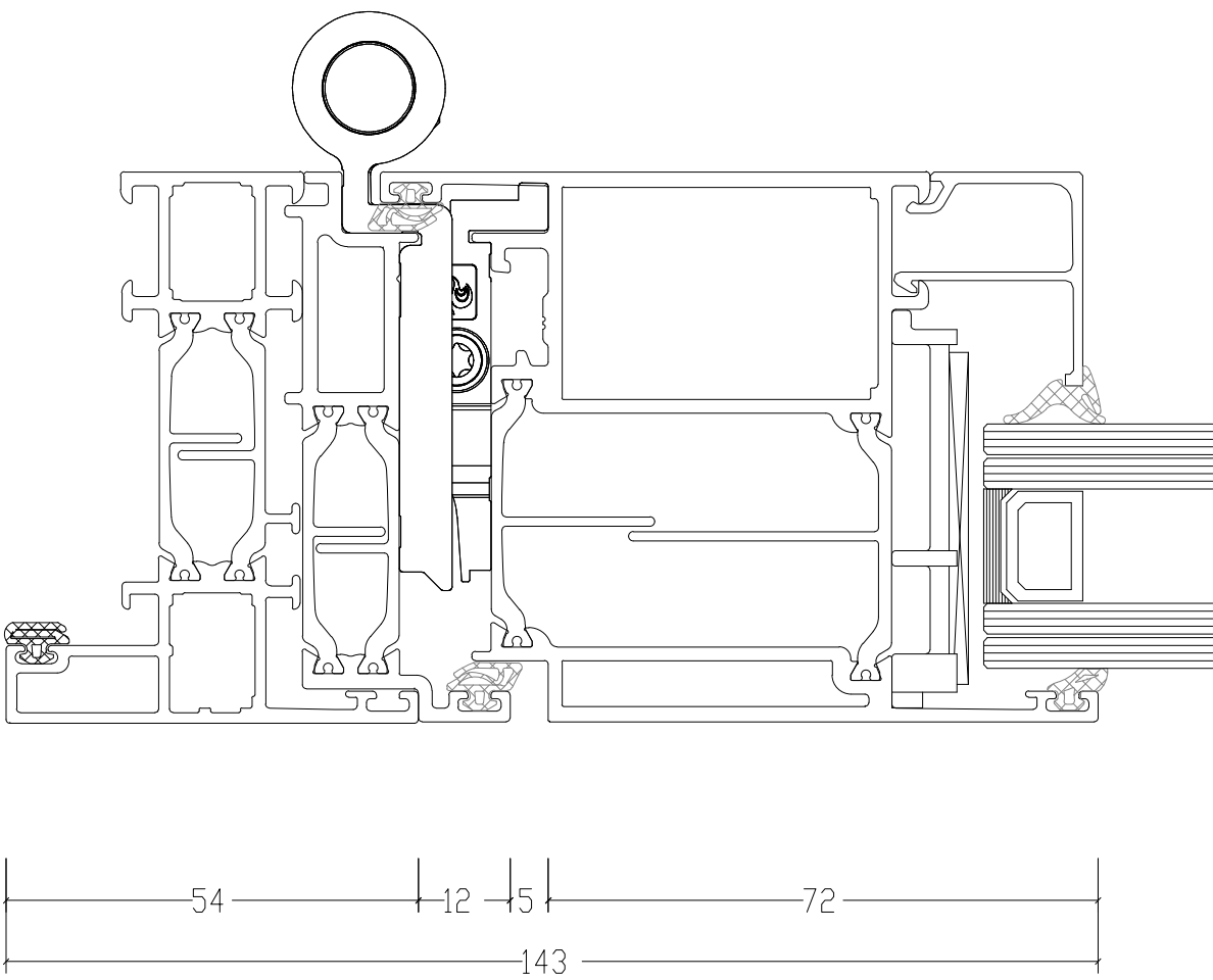
DUBBEL GLAS
