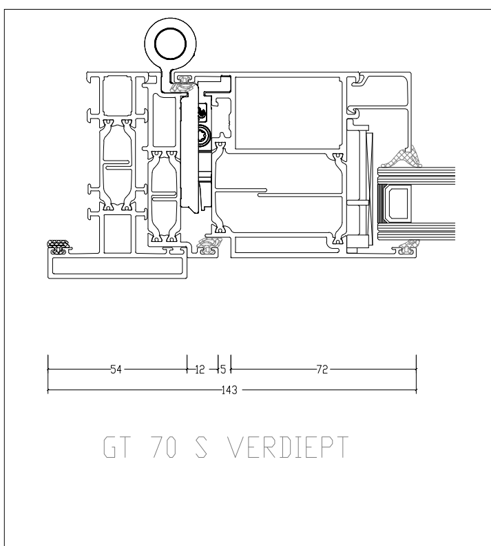
VARIATIES UITVOERING 1:2
