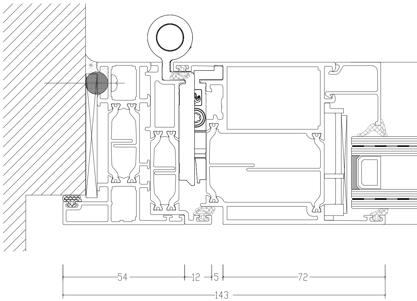
BOUWKUNDIGE AANSLUITINGEN 1:1
