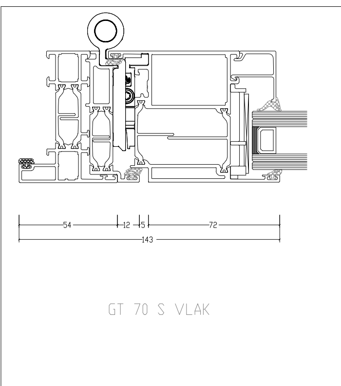
VARIATIES UITVOERING 1:2
