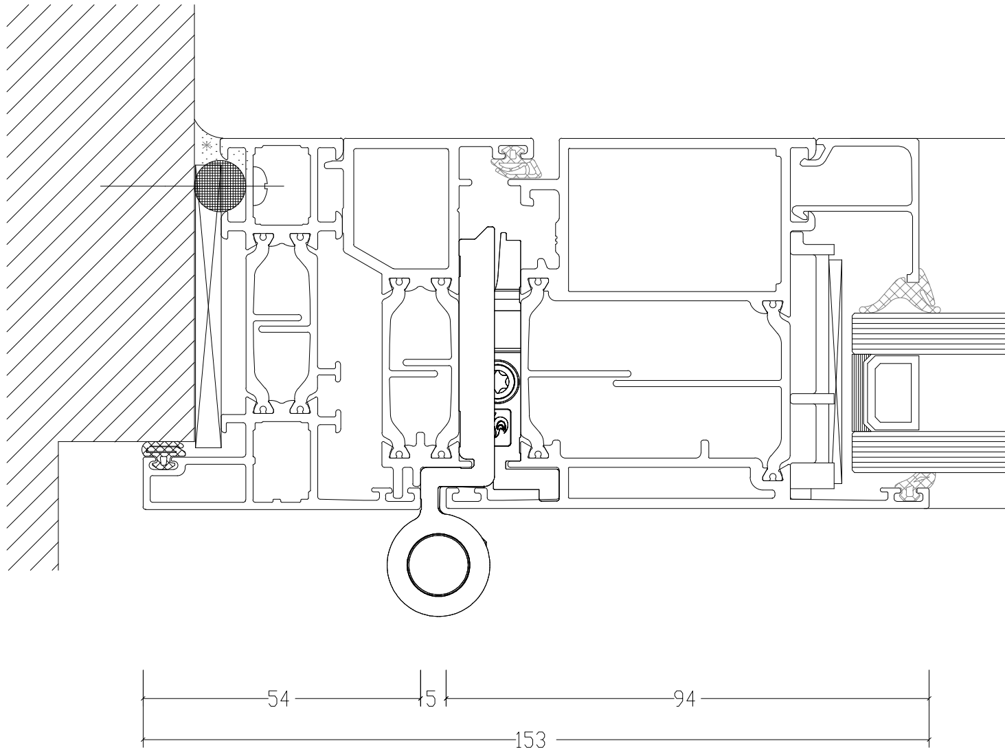
BOUWKUNDIGE AANSLUITINGEN 1:1
