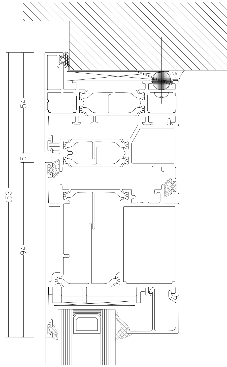
AANSLUITING BOVEN
