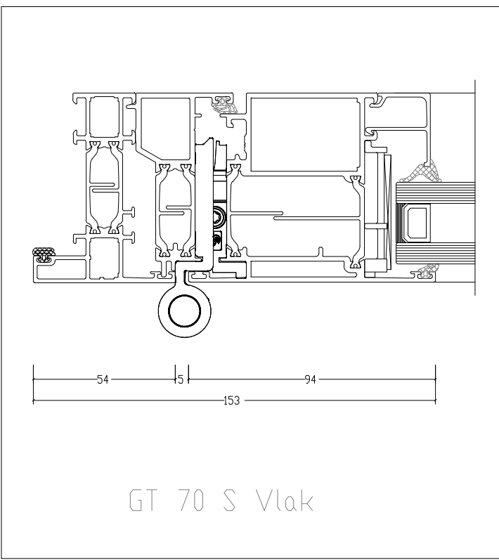
VARIATIES UITVOERING 1:2
