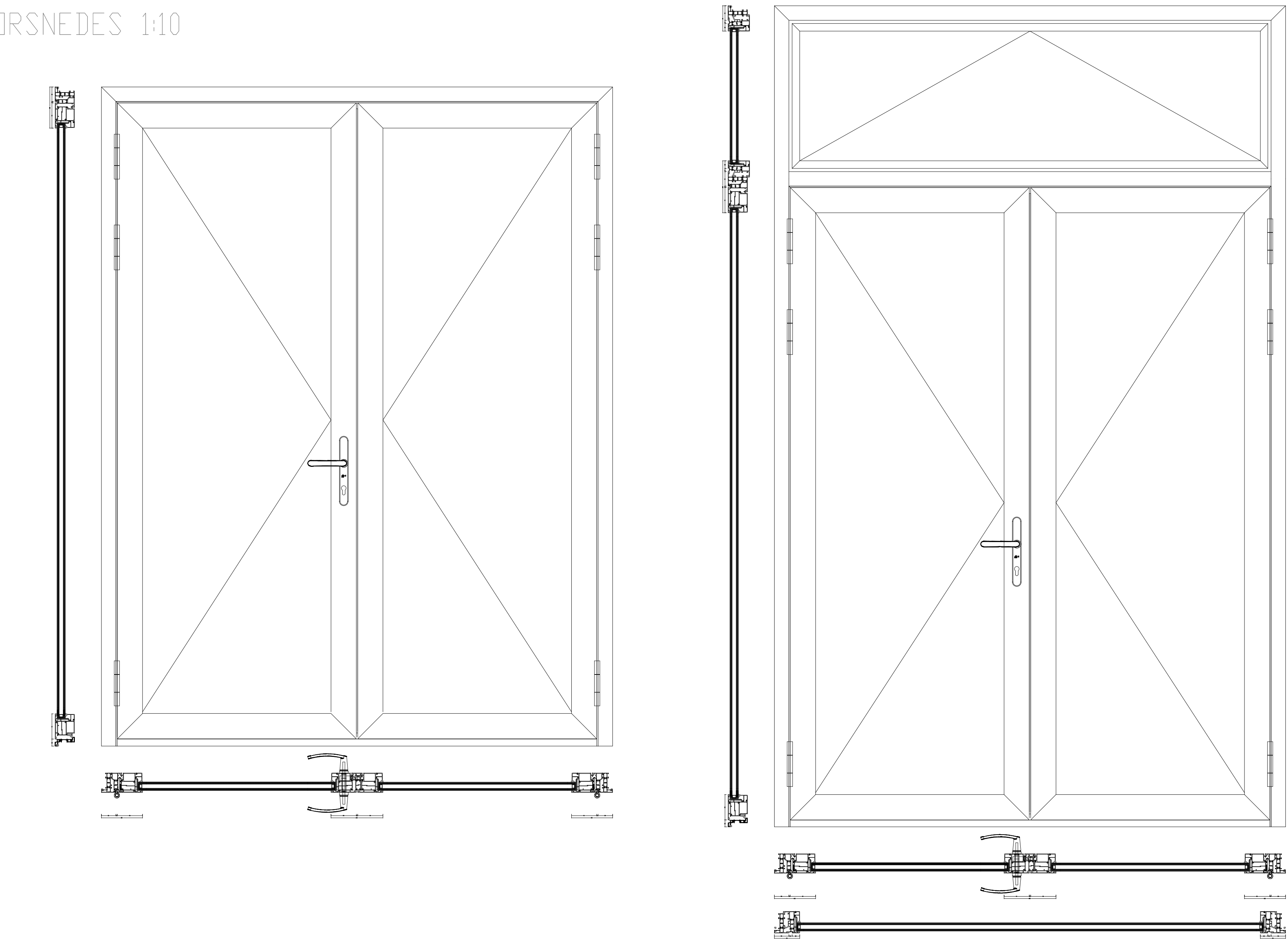
DUBBELE DEUR
