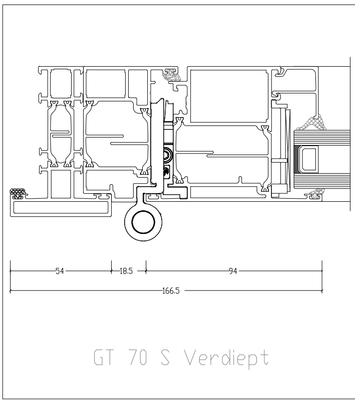
VARIATIES UITVOERING 1:2
