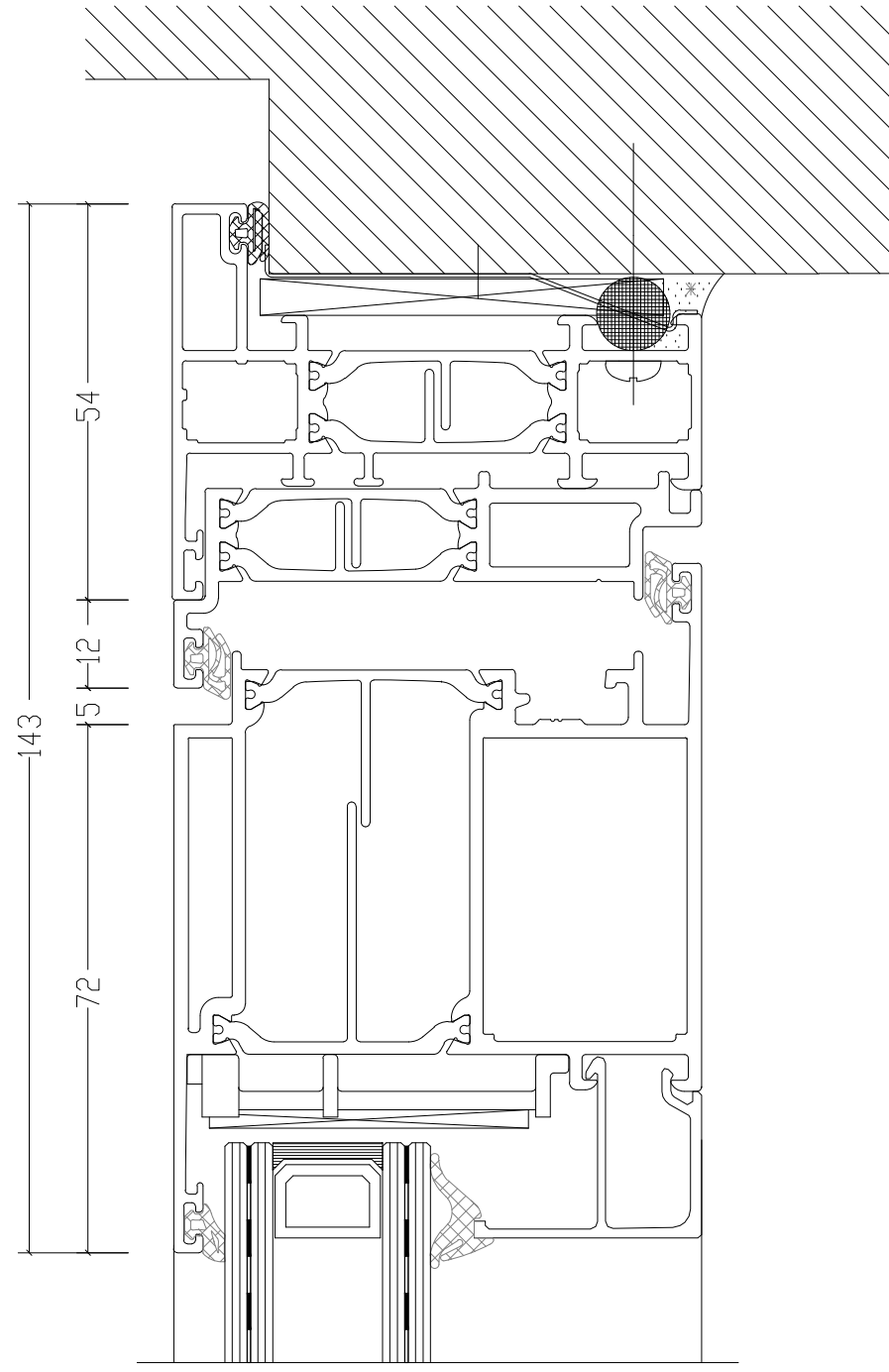
AANSLUITING BOVEN
