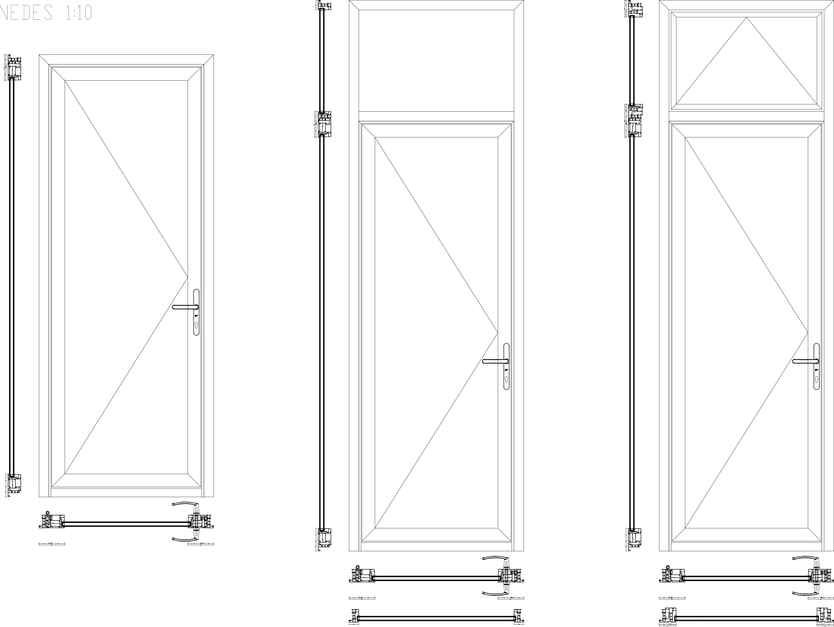
ENKELE DEUR
